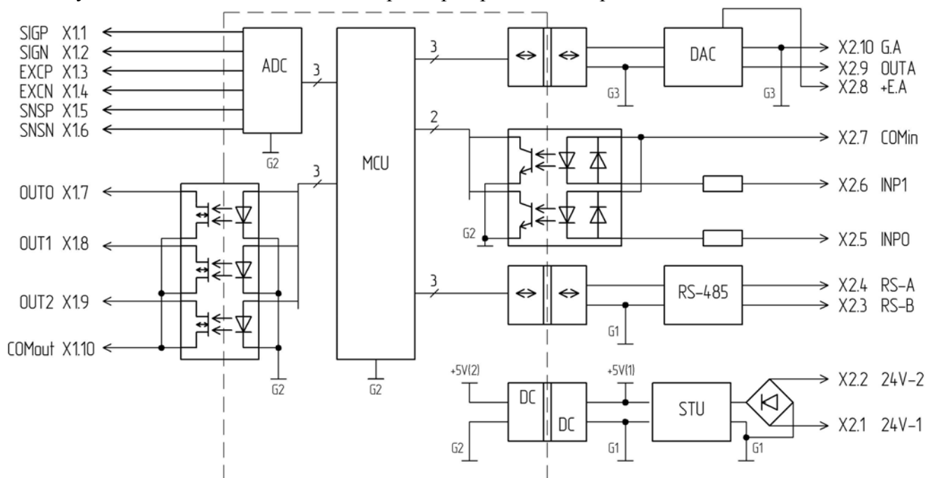
Рис. 2. Функциональная схема тензоКонтроллера
