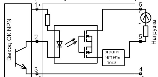
PSA-NPN-D (NPN в сухой контакт, гальв. развязанный)
