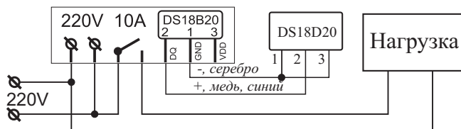
Рис.1. Схема подключения с двухпроводным датчиком. Применяется при длине провода датчика не более 2-3 м.
