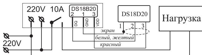
Рис.2. Схема подключения с трехпроводным датчиком. Применяется при длине провода датчика более 2-3 м.
