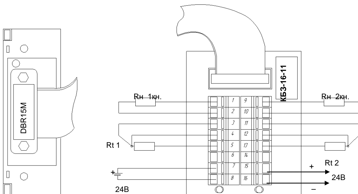
Рисунок 2.3 - Схема внешних соединений БПО-32
