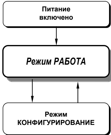
Рисунок 4.1 - Диаграмма режимов работы и настройки индикатора ИТМ-112
