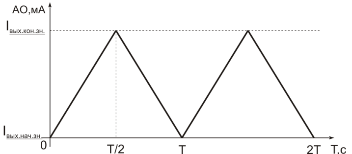
Рисунок 7.11.1 – Диаграмма аналогового выходного сигнала
