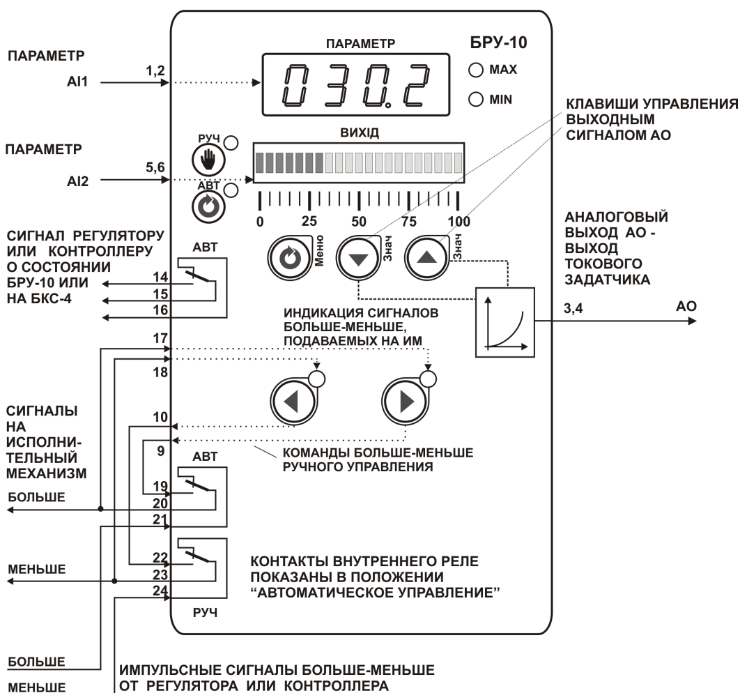
Рисунок 7.8.1 - Блок-схема режима 7
