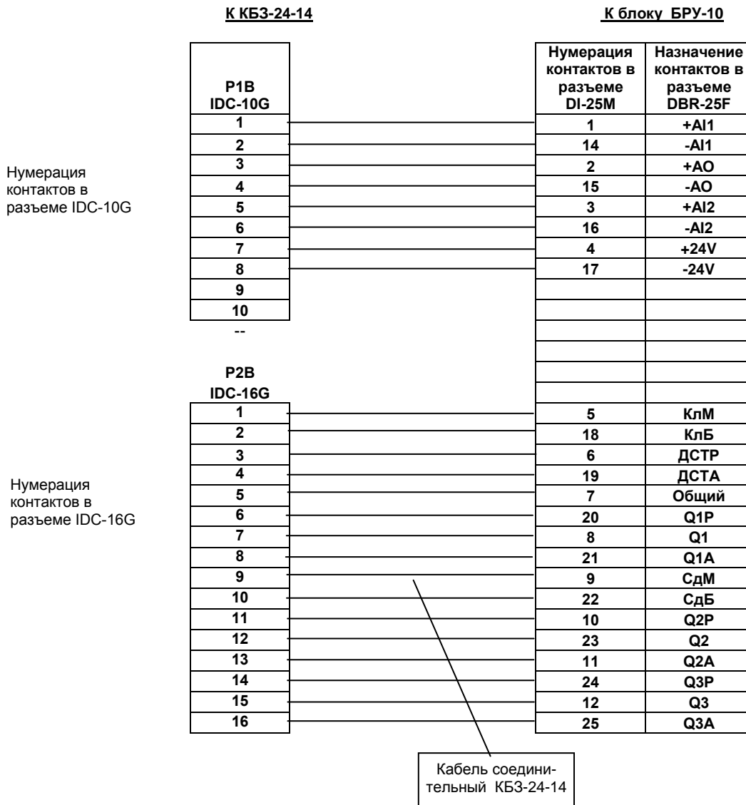
Рисунок Б.8 - Схема проколки кабеля клеммно-блочного соединителя КБЗ-24-14-0,75
