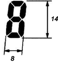
Размеры индикаторов (дисплея): ПАРАМЕТР
