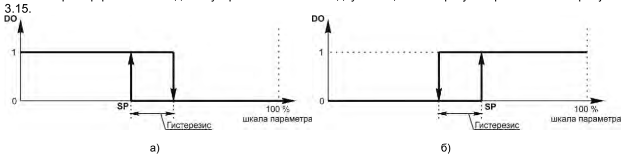
Рисунок 3.15 – Пример работы выходного устройства: а) по логике обратного 2-х позиционного управления п. CTRL.00=0000, п. CTRL.01=0000, б) по логике прямого 2-х позиционного управления п. CTRL.00=0000, п. CTRL.01=0001
