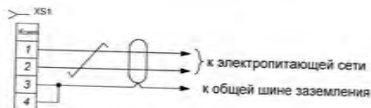
XS1 - соединитель ОНЦ-РГ-09-4/14-Р12 (2РМ14КПН4Г1В1)
