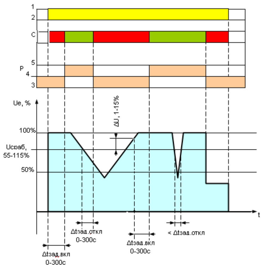
Рисунок 5 - Диаграмма работы реле НЛ-18-2
