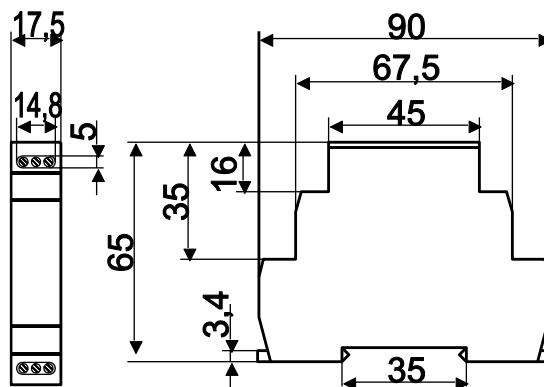
Рисунок 1 - Габаритные и установочные размеры реле
