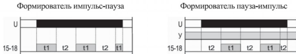
Рисунок 5 - Функциональные диаграммы работы
