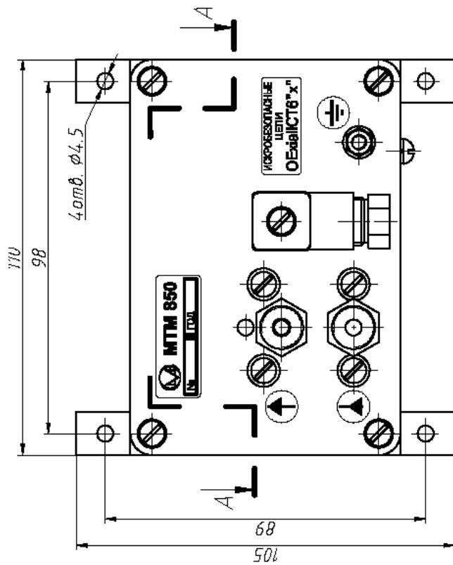
Рисунок 1 – Внешний вид и устройство переключателей
