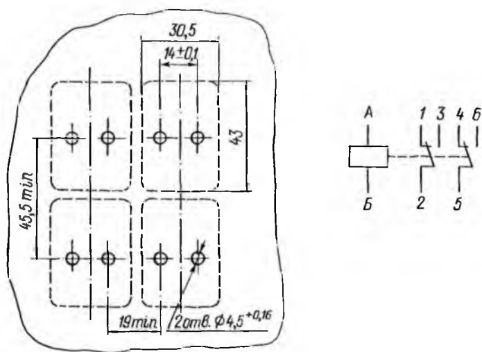
Рис. 2-78. Разметка для крепления и принципиальная электрическая схема
