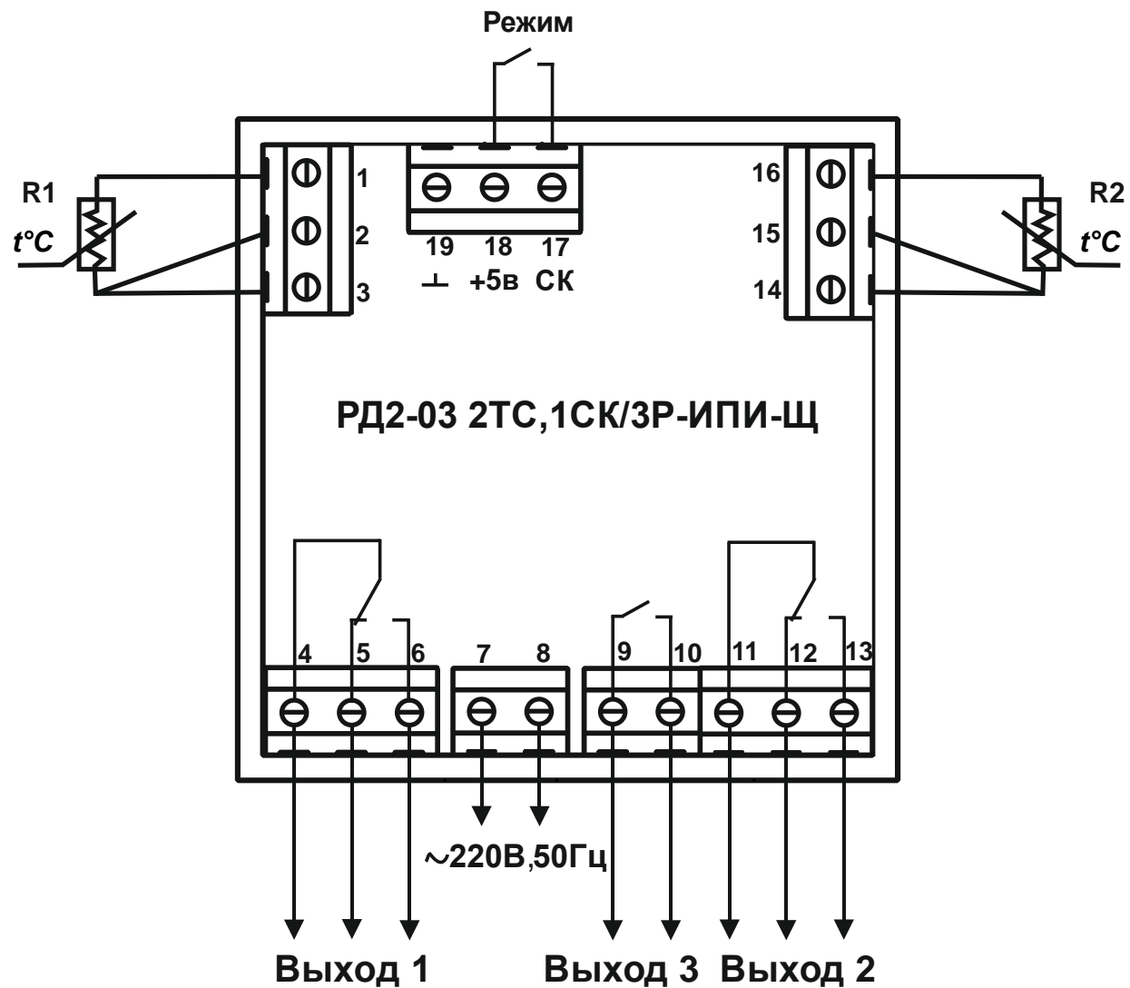
Рисунок 8.1 – Схема подключения ТС, интерфейса связи RS-485, источника питания и исполнительных устройств
