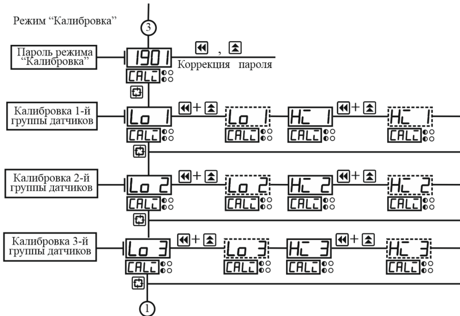
Ри- сунк 3.21 – Схема алгоритма работы в подрежиме "Калибровка 1-го канала"
