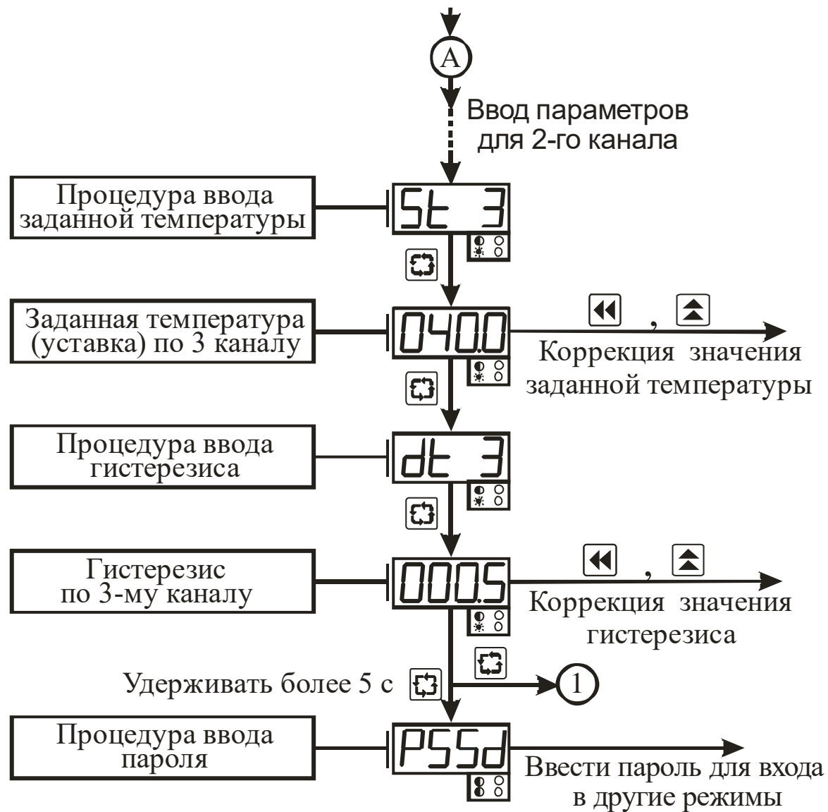
Рисунок 3.4 – Схема алгоритма работы прибора при типе логики работы выхода “01” и “02” (окончание)
