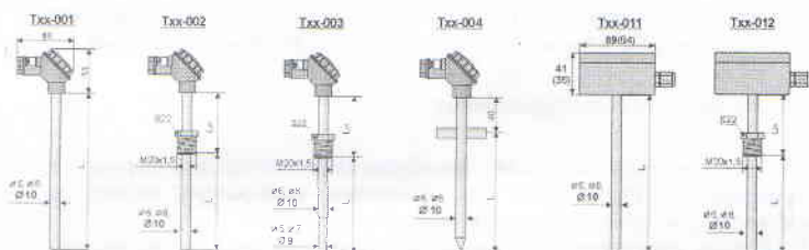
Рисунок 3 - Группа 0. Преобразователи погружаемые
