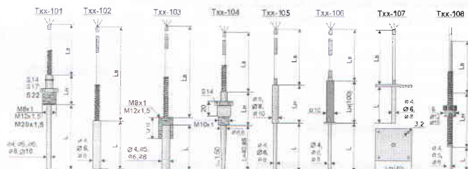
Рисунок 4 - Группа 1. Преобразователи погружаемые с кабельными выводами
