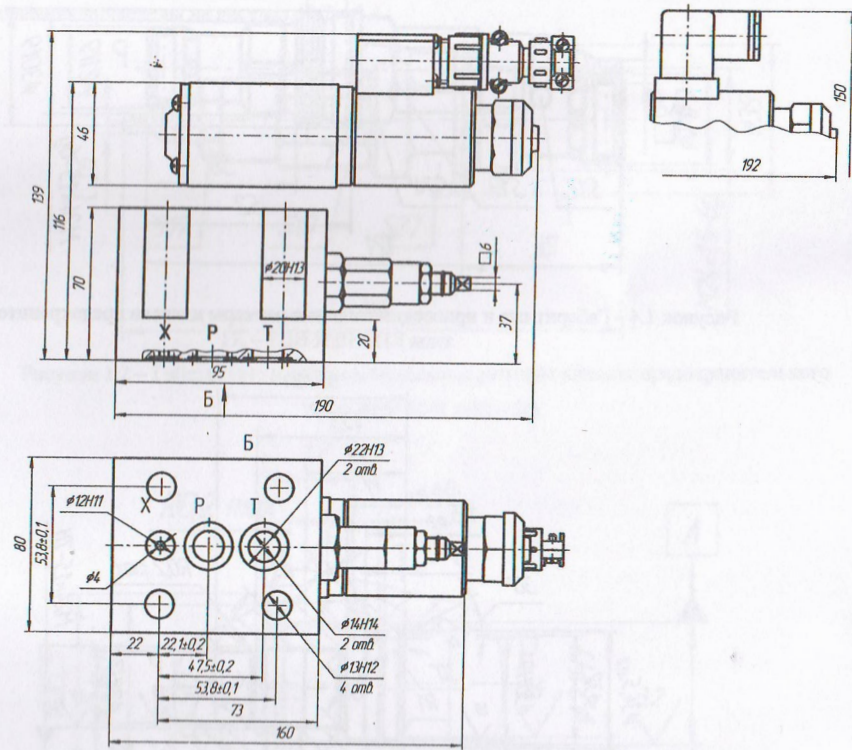
Рисунок 1.4 - Габаритные и присоединительные размеры клапана предохранительного типа КПР 10/X CXX - XX
