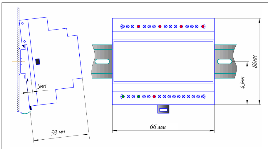
Рис.2 Общий вид.
