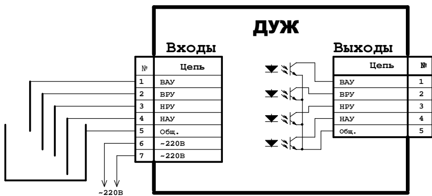
Рис.1. Схема подключения.
