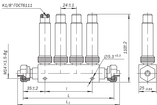
Рис.1. Блок дросельный смазочный БДИ
